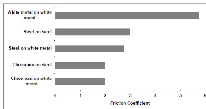
شکل (۱) ضریب اصطکاک فلزات مختلف در تماس با یکدیگر (منبع) (Bzar11)
